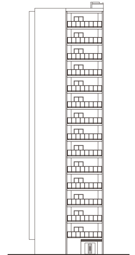
東立面図
