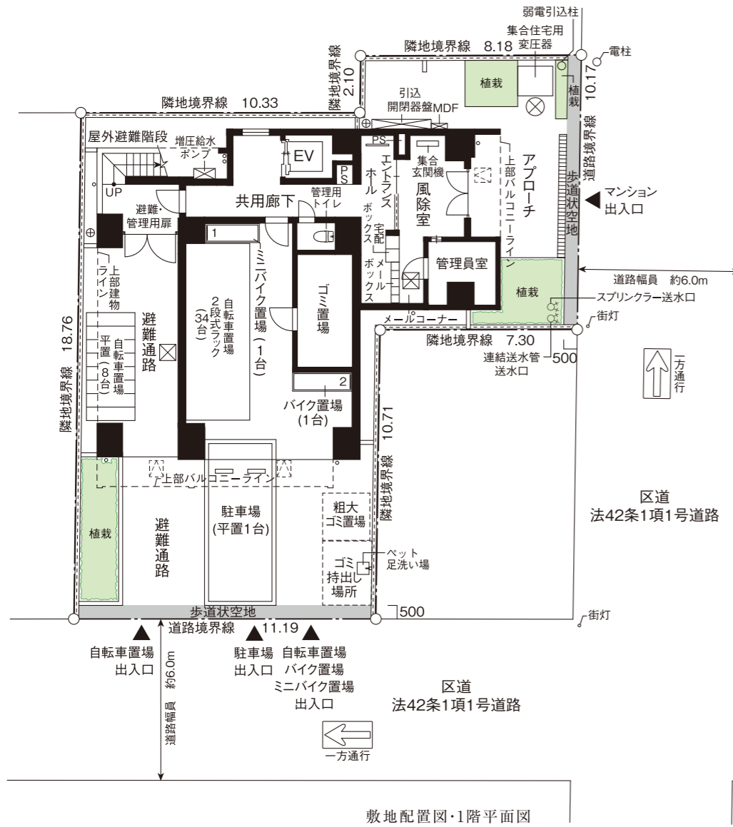
敷地配置図・1階平面図
