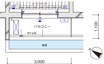
●101号室部分図
