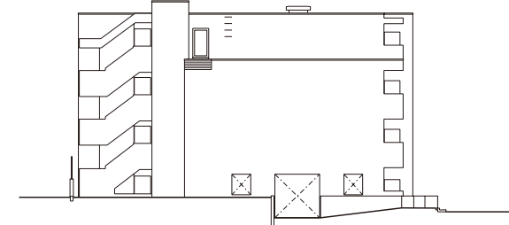
東側立面図
